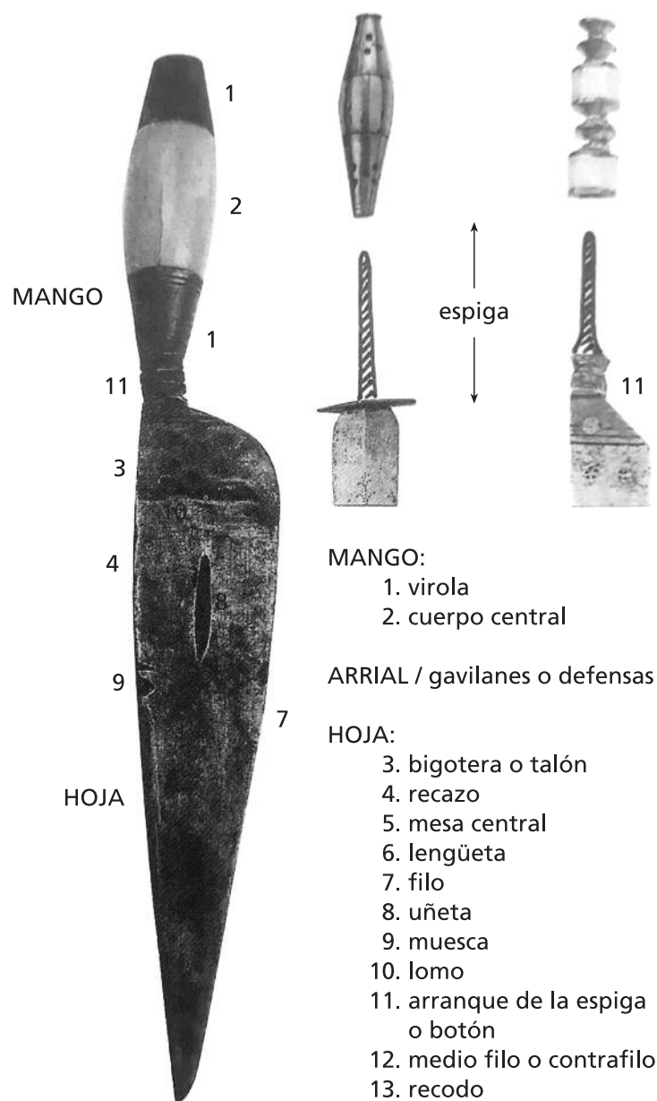
Cuchillo de Albacete tipo B. Siglo XIX. (La cuchillería de Albacete. Sánchez Ferrer. 2005).
