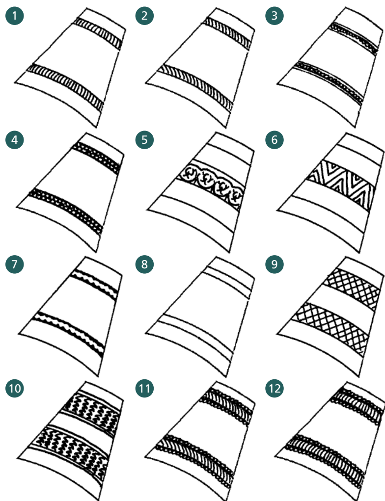
Dibujo de las diferentes tipologías de los casquillos del siglo XIX y principios del XX. Elaboración propia.
